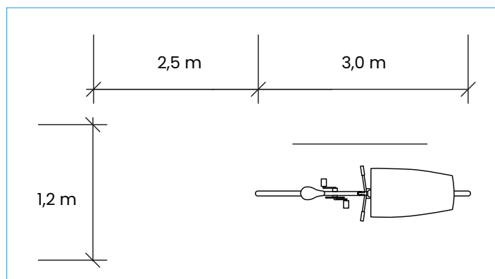
Figure 50 Dégagements à prévoir pour des vélos plus long ou large
