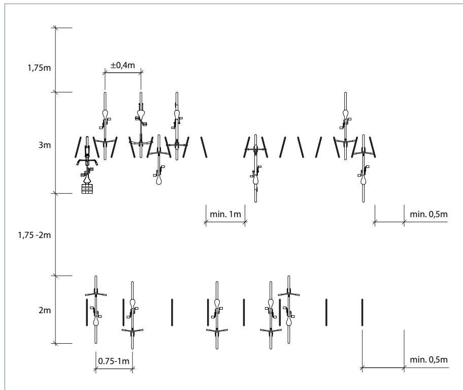
Figure 49 Dégagements à prévoir pour des vélos standard
