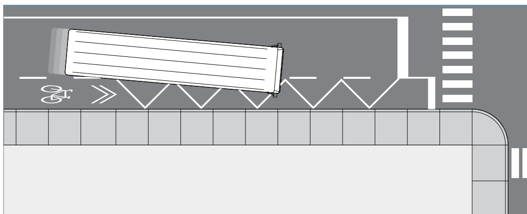
Figure 56 Débarcadère pour autobus situé en bordure de trottoir qui empiète sur la voie cyclable
