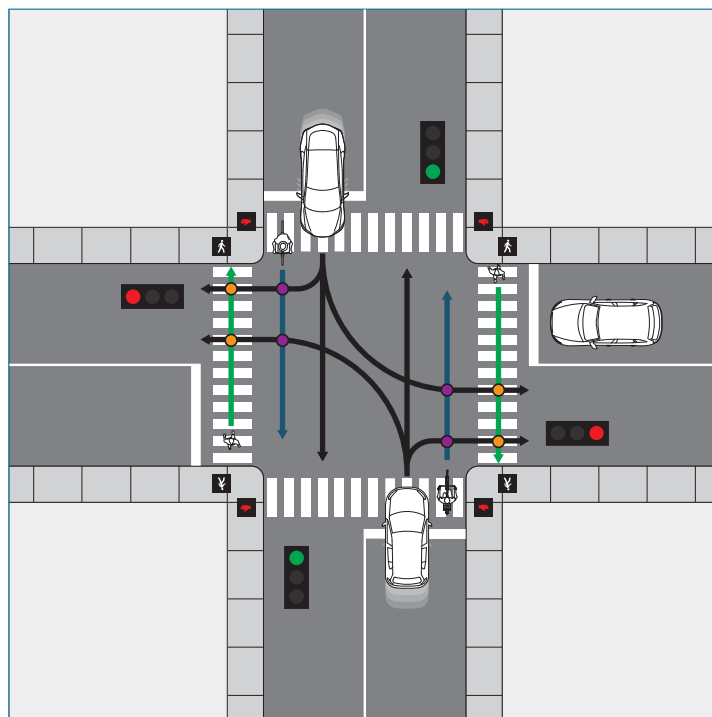
Figure 14 Phase piétonne non protégée
