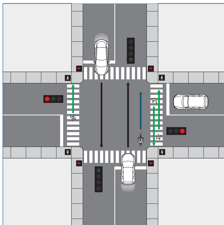
Figure 15 Phase piétonne protégée
