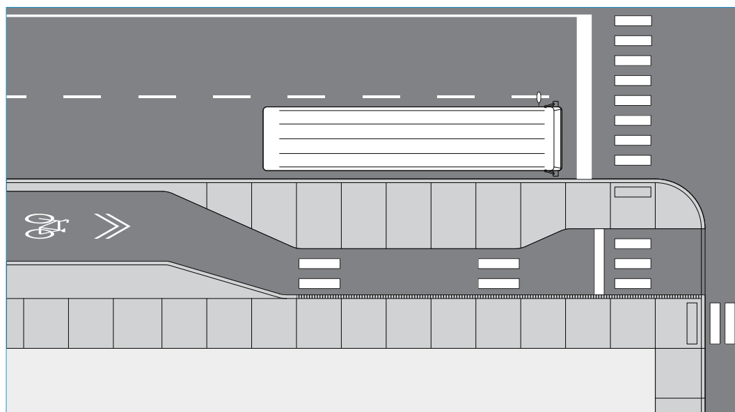
Figure 54 Débarcadère pour autobus dans la voie de circulation
